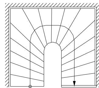
Typ H
