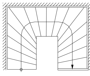
Typ H
