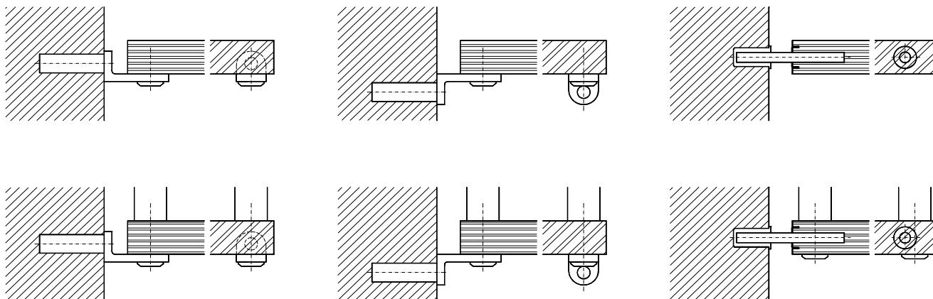
Wandanker: Winkel
